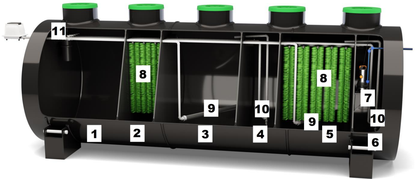
Рис. 3 Устройство станции «Диамант 25».
