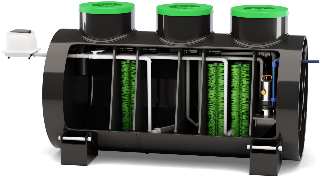
Рис.1 Устройство станций Диамант моделей 3,8.
